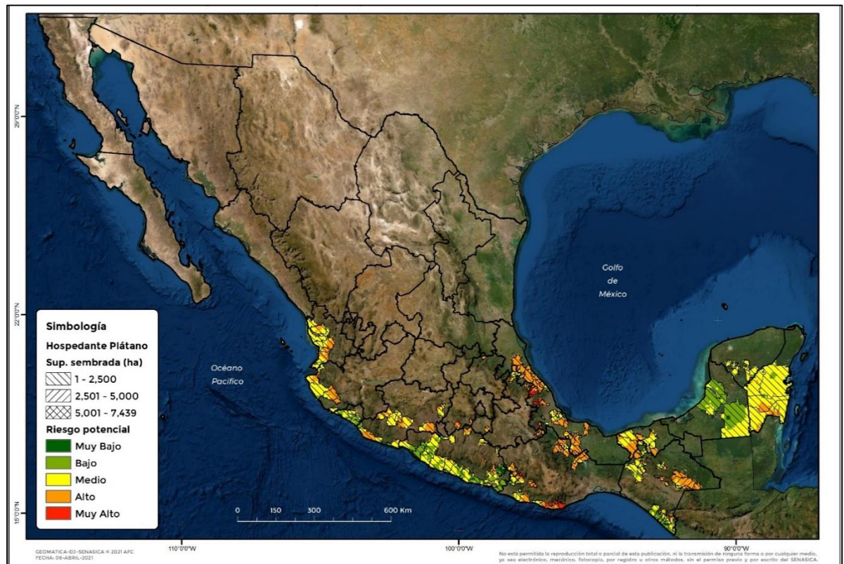
Figura 3. Proyección de condiciones climáticas óptimas para el potencial establecimiento de Foc R4T .
