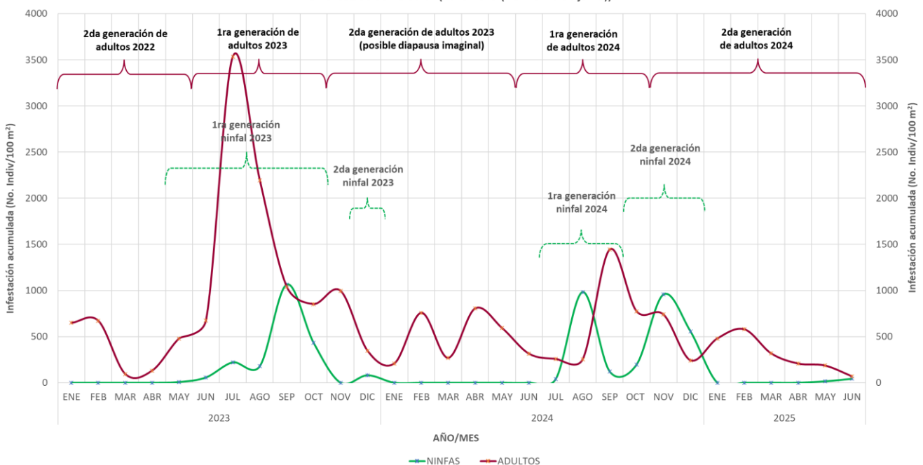
Dinámica Poblacional de los Estados Biológicos de la Langosta Centroamericana en el estado de Veracruz (2023-2025 (Del 1 al 20 de junio))
